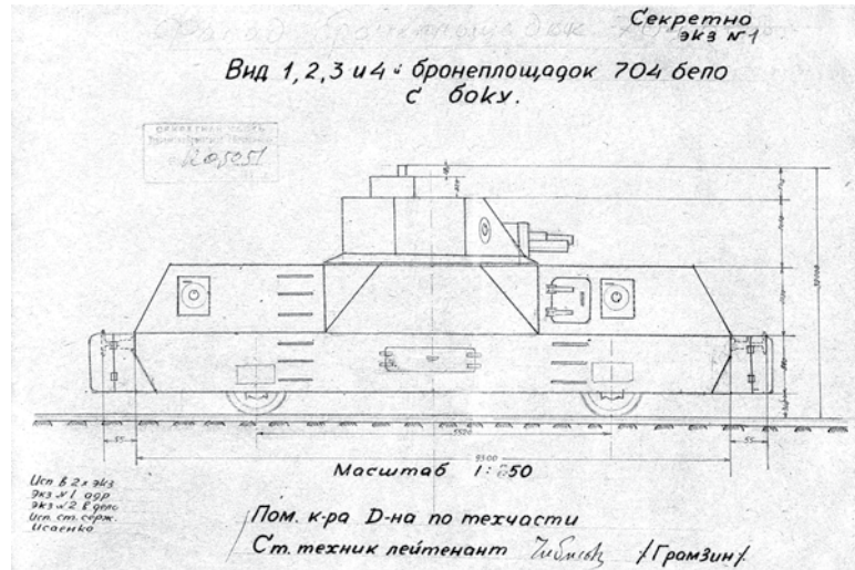
Чертежи бронеплощадки бронепоезда «Лунинец»
