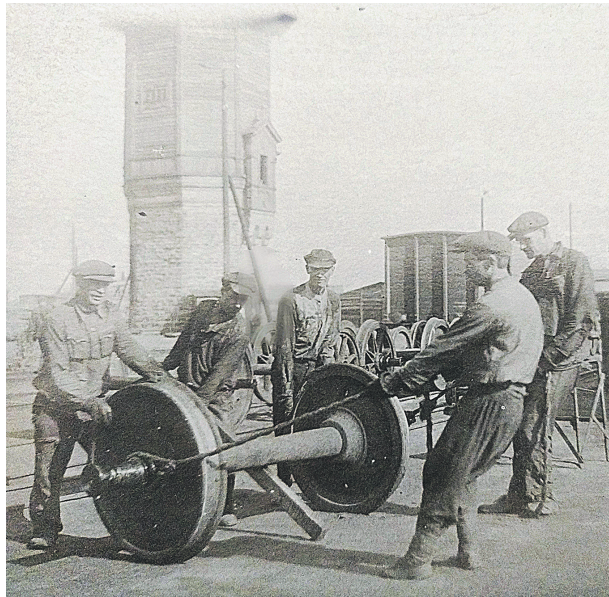
Доставка при помощи «карандаша» и веревок колесной пары. Цех по ремонту грузовых вагонов вагонного участка №3 станции Болотная, 1940-е гг. Фото из фондов МККУ «Болотнинский районный историко-краеведческий музей»
